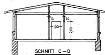
SCHNITT C-D
