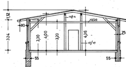
SCHNITT A-B
